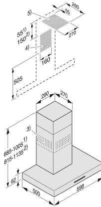
DA 416-6, DA 416-7 (Installation drawing)
